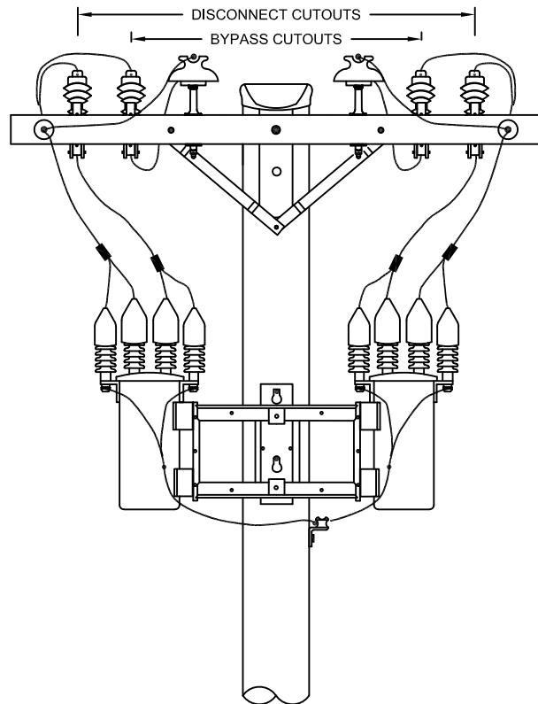
LOAD SIDE
