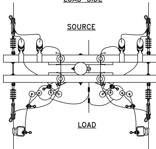
LOAD SIDE
